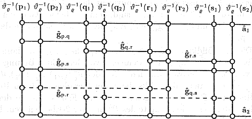
Abbildung 4. Geradenkonfiguration im \bar{E}^3 (Schema)
