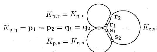
Abbildung 5. Entartete Büschelsatz-Konfiguration.
