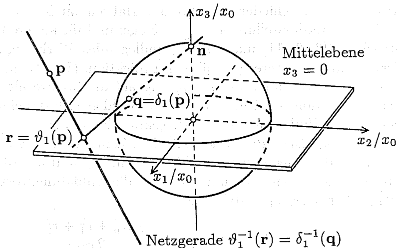
Abbildung 2. Verallgemeinerte stereographische Projektion \delta_1
