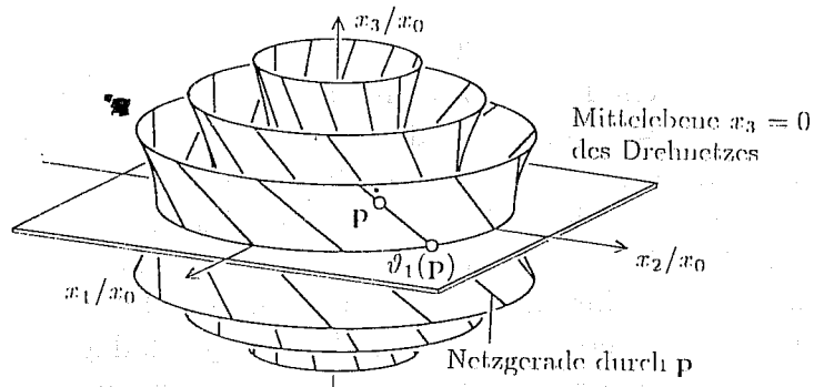
Abbildung 1. Netzprojektion \vartheta_1
