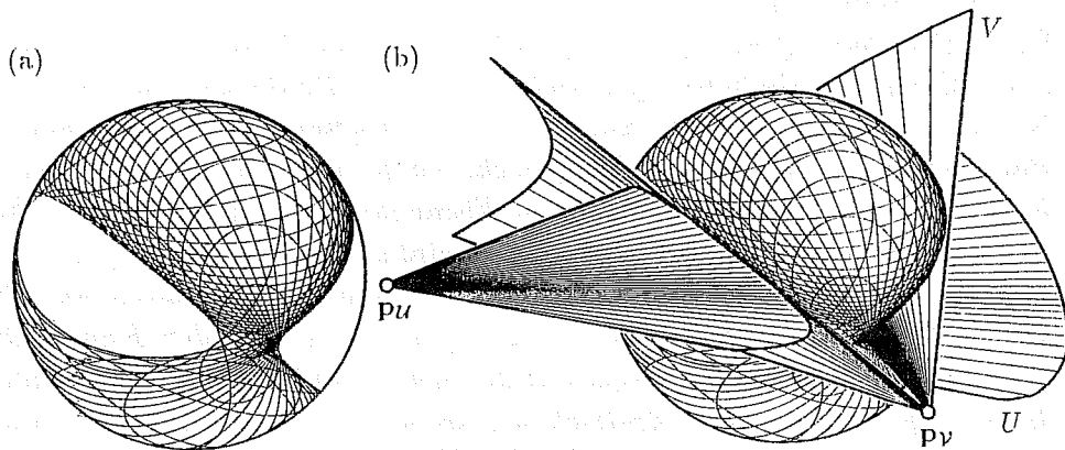
Abbildung 6. Biquadratische Parameterdarstellung der Kugel
