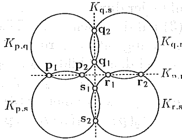
Abbildung 3 Büschelsatz-Konfiguration
